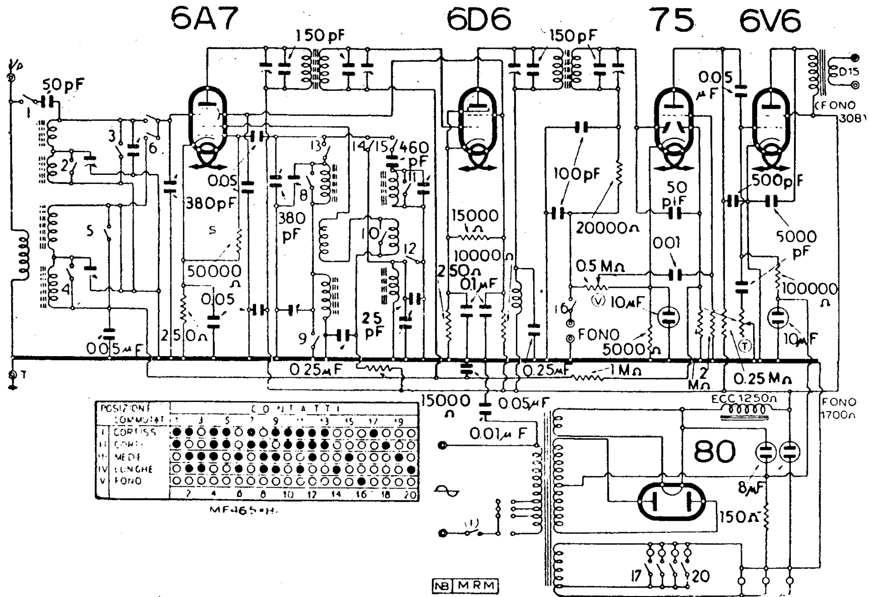
WATT RADIO - MOD. «SABAUDO II»
